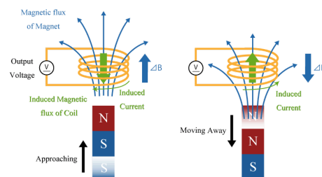
Imagen 1. Representación de sensor magnético Coiled
